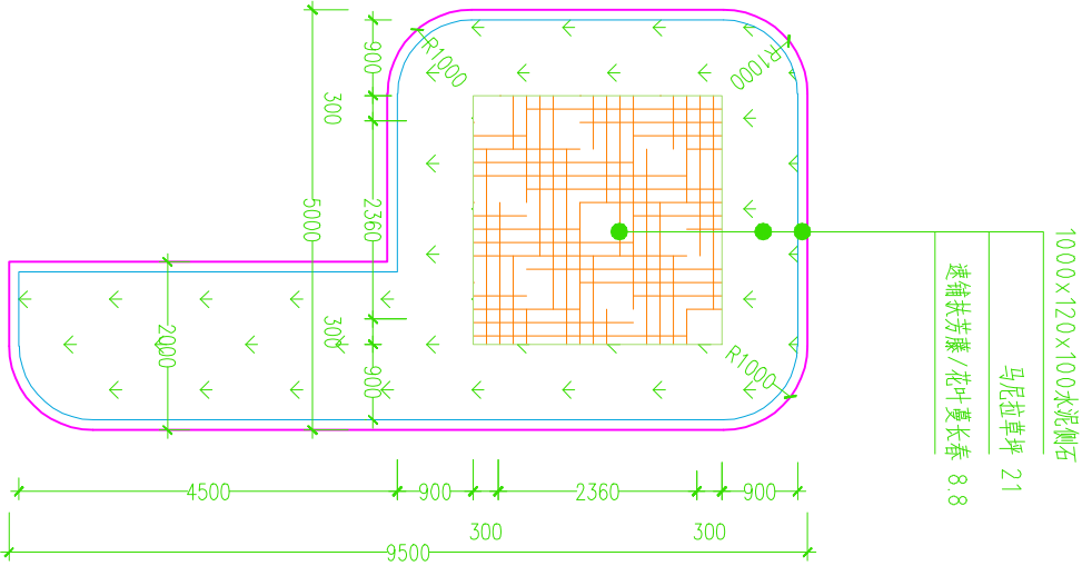
侧方停车区域 1:100 面积约33m 2 共6块
